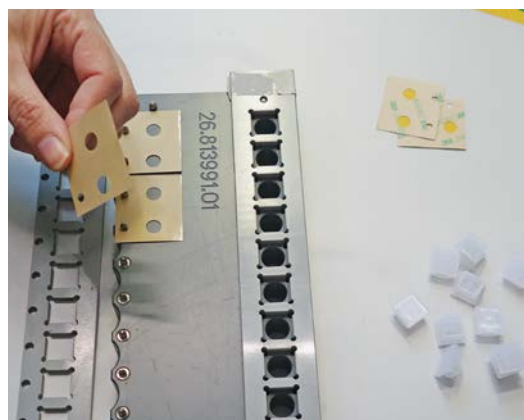
Une pièce estampée dans un adhésif double face est utilisée pour assembler le bouton poussoir (blanc) et le cache en laiton de l'interrupteur.
