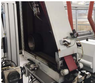
Vollautomatische Maschine bestückt mit 3M Schleifband
